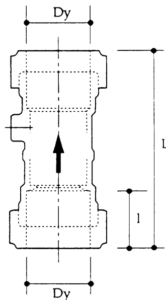
TYP IND-188-CRM Anslutning med klämringskoppling.
